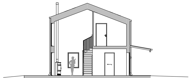
SEKTION
