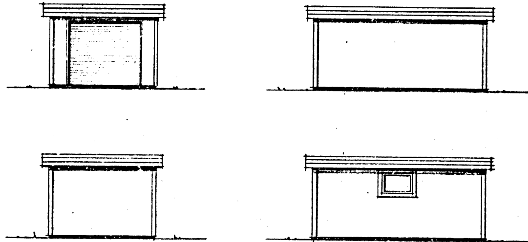
FASADER 1:100
