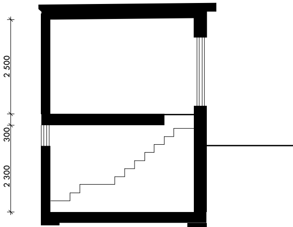
TYPSEKTION
