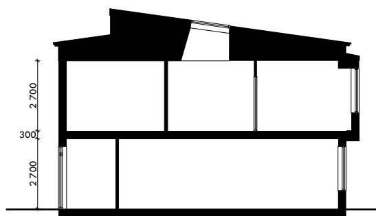
TYPSEKTION
