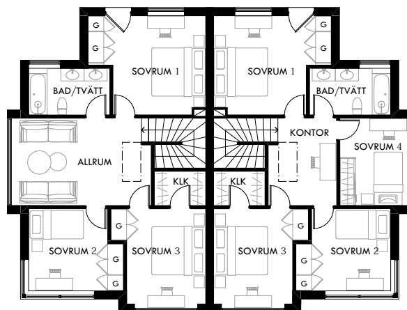
ÖVRE PLAN
