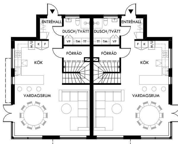
ENTRÉPLAN
